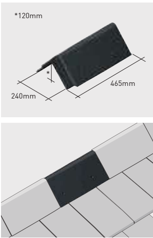
Q91*K | Piramide vorst
