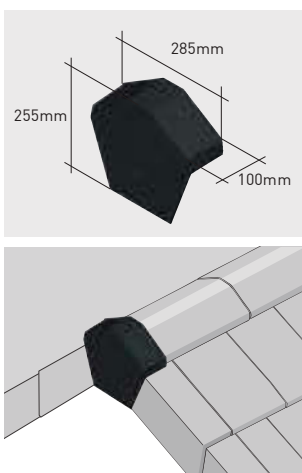
Q124*K | Begin- eindkapje
