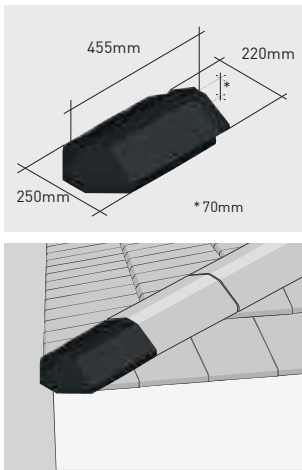
Q122*K | Hoekkeper beginvorst
