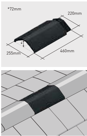
Q120*K | Hoekkepervorst Nederlands model
