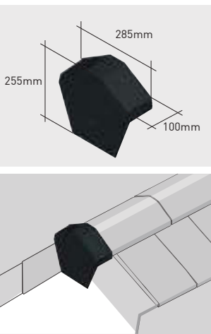
Q147*K | Begin- eindkapje
