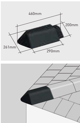
Q109*K | Hoekkeper beginvorst
