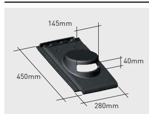
Q87*K | Planum doorvoerpan
