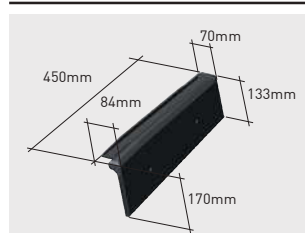
Q88*K | Planum rechter gevelpan
