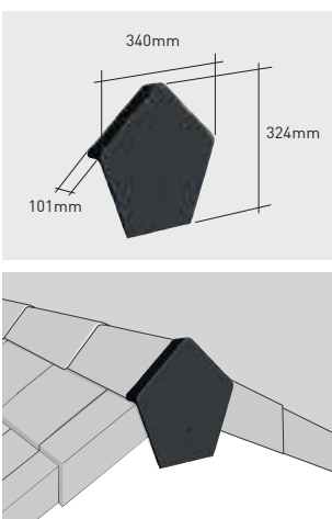
Q92*K | Begin- eindkapje
