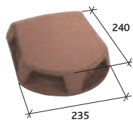
Lanterne bi-section Ø 120 utile et Ø 150 utile (Section d'aération : 130 cm 2 ) Réf. 1000
