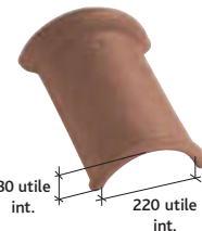
Faitière 1/2 ronde à emboîtement (2,5 au ml) Réf. 717
