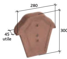
Fronton pour faitière losangée à recouvrement Réf. 809
