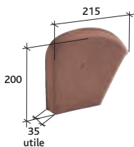
Fronton gauche pour faitière Shed Réf. 806
