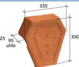
Fronton de rive universelle Réf. 1080
