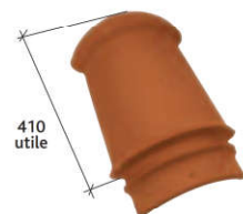
About d'arêtier 1/2 rond à emboîtement Wardrecques (2)(6) Réf. 862
