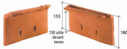
Rive individuelle gauche à recouvrement Monopole N°1 (4,2 au ml) Réf. 306.42
