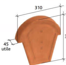
Fronton pour faîtière 1/2 ronde à recouvrement Réf. 807
